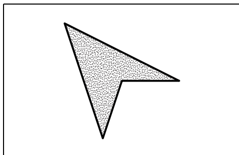
Рис. 52. Невыпуклый четырёхугольник.
