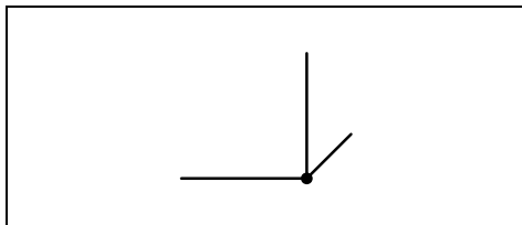
Рис. 156. Вершина куба.
